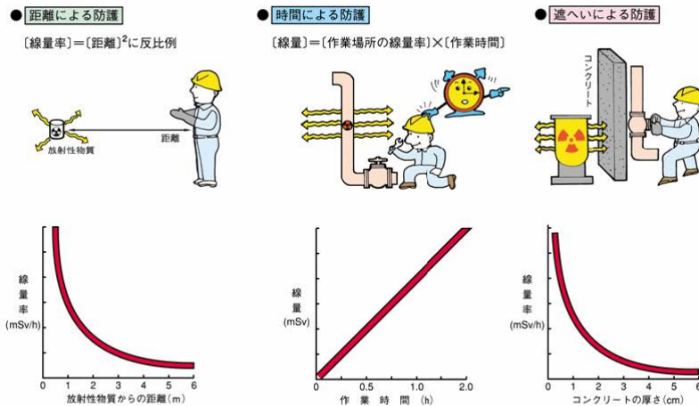
図1 遮へい3原則の図
